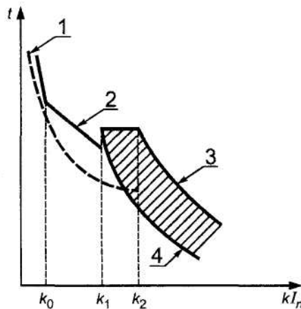
Рисунок 1 — Примерная диаграмма проверки времятоковой характеристики по результатам испытаний при «пороговых» токах
