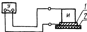
У - установка; И - испытуемое изделие; 1 - металлическая пластина; 2 - пластина из диэлектрического материала
