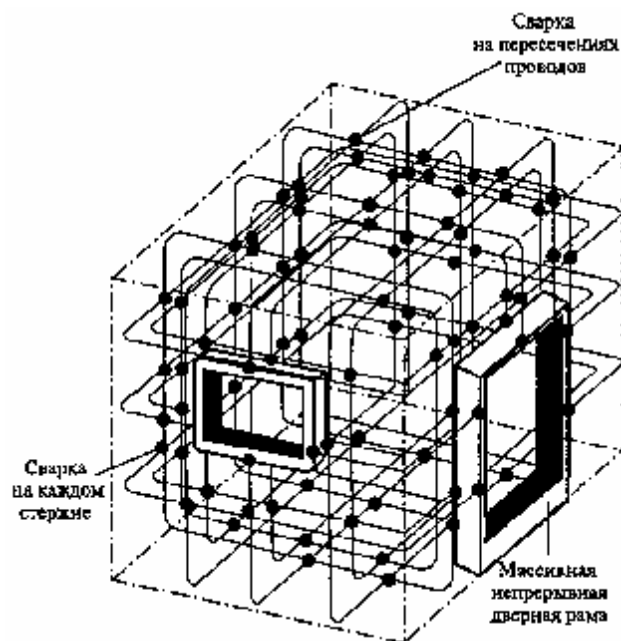
Рис. 4.3. Пространственный экран из стальной арматуры
