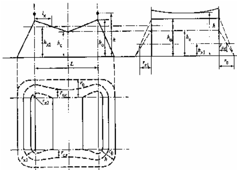
Рис. 3.4. Зона защиты двойного тросового молниеотвода
