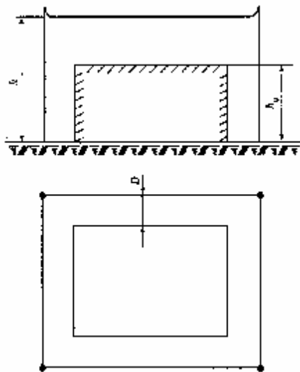
Рис. 3.5. Зона защиты замкнутого тросового молниеотвода
