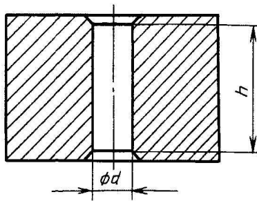
Рисунок 4 - Калибр для проверки на соосность (см. 5.4)
