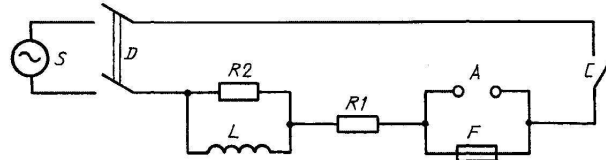
Рисунок 5 - Типовая схема для испытаний на отключающую способность плавких вставок с высокой отключающей способностью (см. 6.3)
