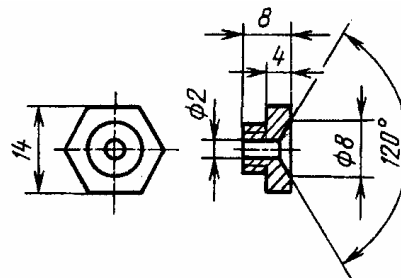
Рисунок 2 - Цоколь для испытания плавких вставок размером 6,3×32 мм. Номинальные токи св. 10 А (см. 4.3.1)
