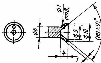
Рисунок 1 - Цоколь для испытания плавких вставок размером 5×20 мм и 6,3×32 мм. Номинальные токи до 10 А включ. (см. 4.3.1)
