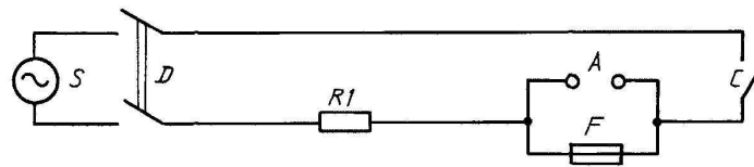
Рисунок 6 - Типовая схема для испытаний на отключающую способность плавких вставок с низкой отключающей способностью (см. 6.3)
